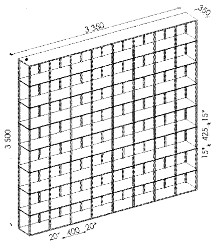
Стелаж книжковий: -металева конструкція труба : 2-2,5*мм RAL9003 стр.
