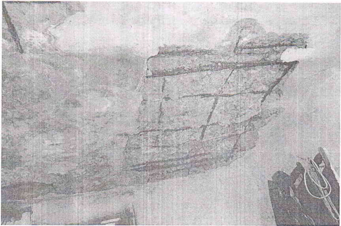
Фото В.9. Приміщення №81, відшарування захисного шару бетону з/б плити перекриття с оголенням кородуючої робочої арматури
