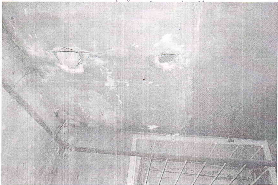
Фото В.10. Приміщення підвалу №83, не проектні отвори, відшарування захисного шару бетону з/б плити перекриття с голенням кородуючої робочої арматури, вісі «17/А-Б»
